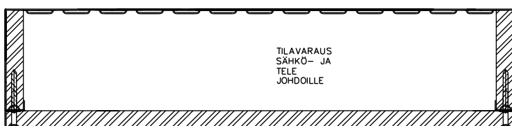
SP.5012 (500*120) EI30 PALOSUOJATTU SÄHKÖJOHTOELEMENTTI ELEMENTISSÄ 465 * 100 TILAVARAUS SÄHKÖ- JA TELEJOHDOLLE PALOERISTYS EI30 PALONSUOJAKIPSILEVY KNAUF DB15 POHJAOSASSA NIPPUSIDELENKIT KAAPELEIDEN KIINNITYSTÄ VARTEN
