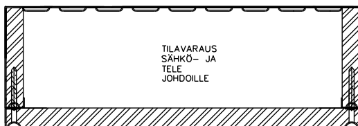
SP.3512 (350*120) EI30 PALOSUOJATTU SÄHKÖJOHTOELEMENTTI ELEMENTISSÄ 315 * 100 TILAVARAUS SÄHKÖ- JA TELEJOHDOLLE PALOERISTYS EI30 PALONSUOJAKIPSILEVY KNAUF DB15 POHJAOSASSA NIPPUSIDELENKIT KAAPELEIDEN KIINNITYSTÄ VARTEN
