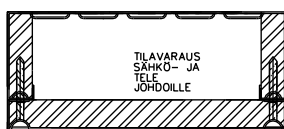
SP.198 (190*80) EI30 PALOSUOJATTU SÄHKÖJOHTOELEMENTTI ELEMENTISSÄ 155 * 60 TILAVARAUS SÄHKÖ- JA TELEJOHDOLLE PALOERISTYS EI30 PALONSUOJAKIPSILEVY KNAUF DB15 POHJAOSASSA NIPPUSIDELENKIT KAAPELEIDEN KIINNITYSTÄ VARTEN
