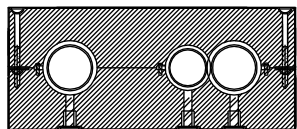
ELEMENTTITYYPPI AS.2812 (280*120) PUTKIKOOT ENINT. KV42 LVK35 LV42
