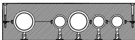
ELEMENTTITYYPPI AS.4312/5 (430*120) PUTKIKOOT ENINT. KV54 LVK35 LV54 LV35/35
