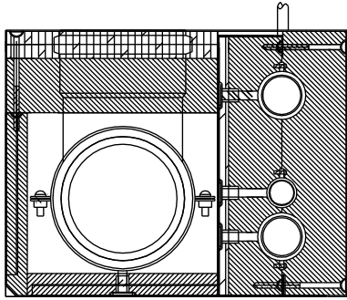
ELEMENTTITYYPPI AS.2431 (245*315) PUTKIKOOT ENINT. V110 KV35 LVK22 LV35 ELEMENTTI NURKKA-ASENNUKSEEN
