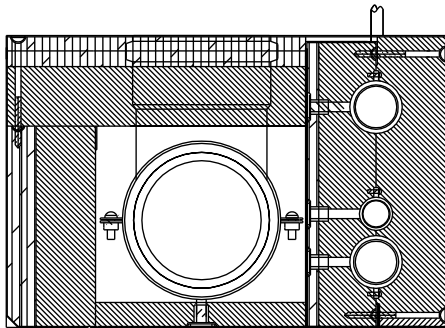
ELEMENTTITYYPPI AS.2437 (245*370) PUTKIKOOT ENINT. V110 KV35 LVK22 LV35 ELEMENTTI VAPAAN SEINÄN ASENNUKSEEN
