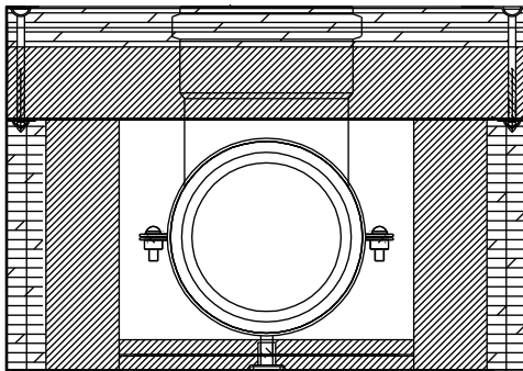
ELEMENTTITYYPPI AS.2435 (245*350) PUTKIKOOT ENINT. V110 ELEMENTTI VAPAAAN SEINÄN ASENNUKSEEN
